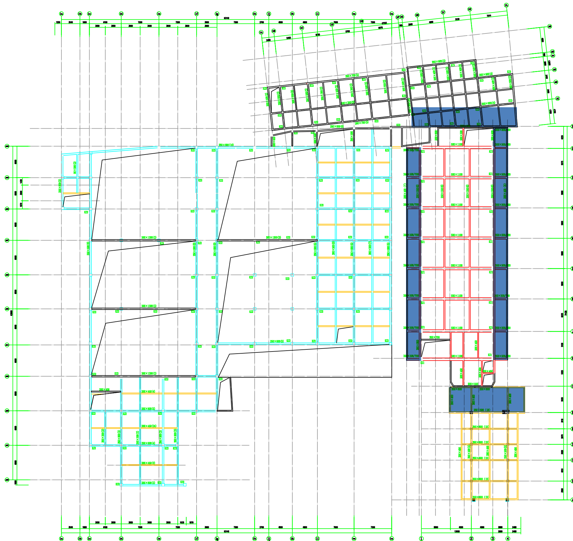
夹层结构平面布置示意图
